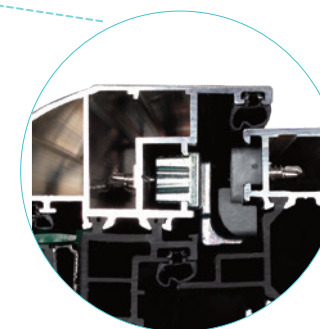
Conçu pour conserver et régler la compression sur la hauteur de l'ouvrant
